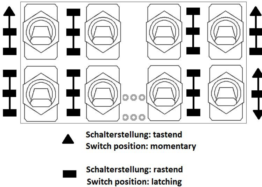
Abb. 3: Empfehlung zur Positionierung der Schaltertypen
